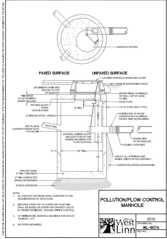
2 POLLUTION/FLOW CONTROL MANHOLE SCALE: N.T.S.
