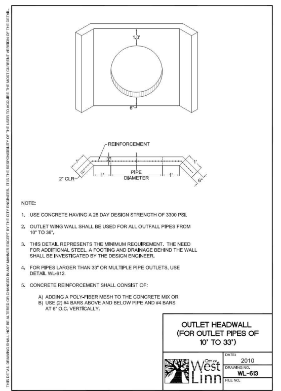
5 HEADWALL SCALE: N.T.S.
