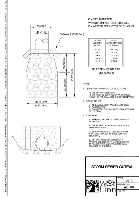
4 STORM SEWER OUTFALL SCALE: N.T.S.
