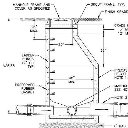
5 STANDARD CLEANOUT (COTG) SCALE: NTS
